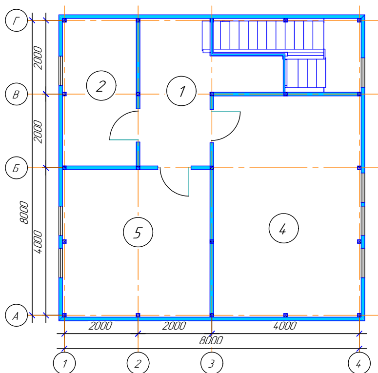
План на відмітці +2,980
