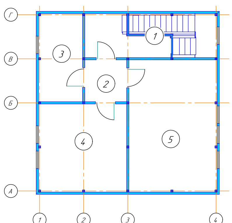
План на відмітці +2,980
