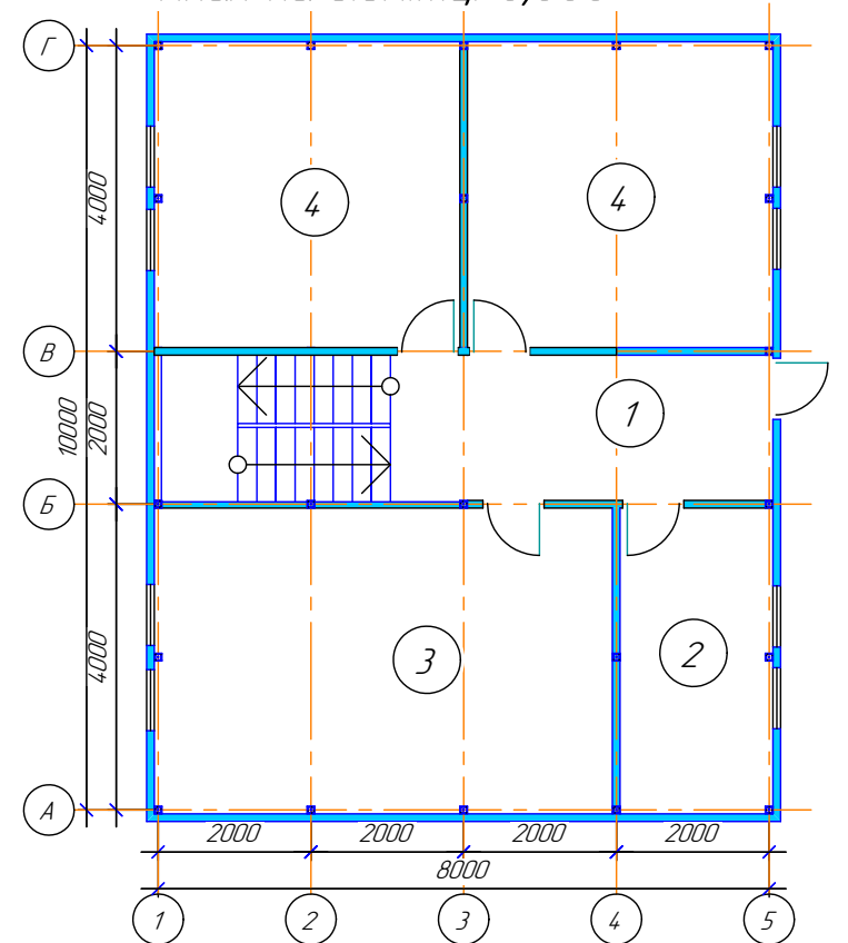
План на відмітці +2,980
