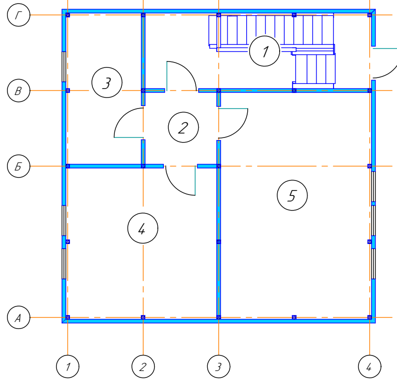
Модель П2 (2-2/2-8/8)
