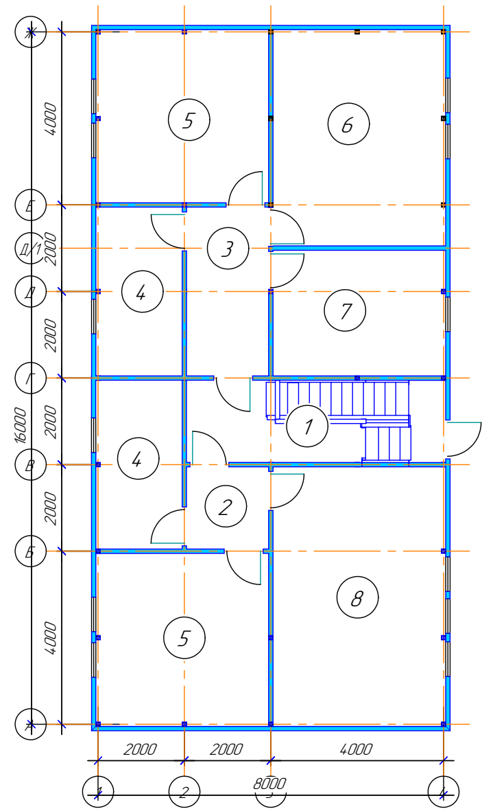
План на відмітці 0,000 та на відмітці +2,980
