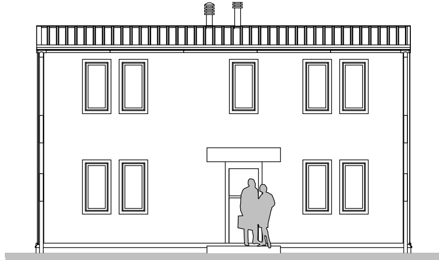
Модель П4 (2-1/6-10/8)
