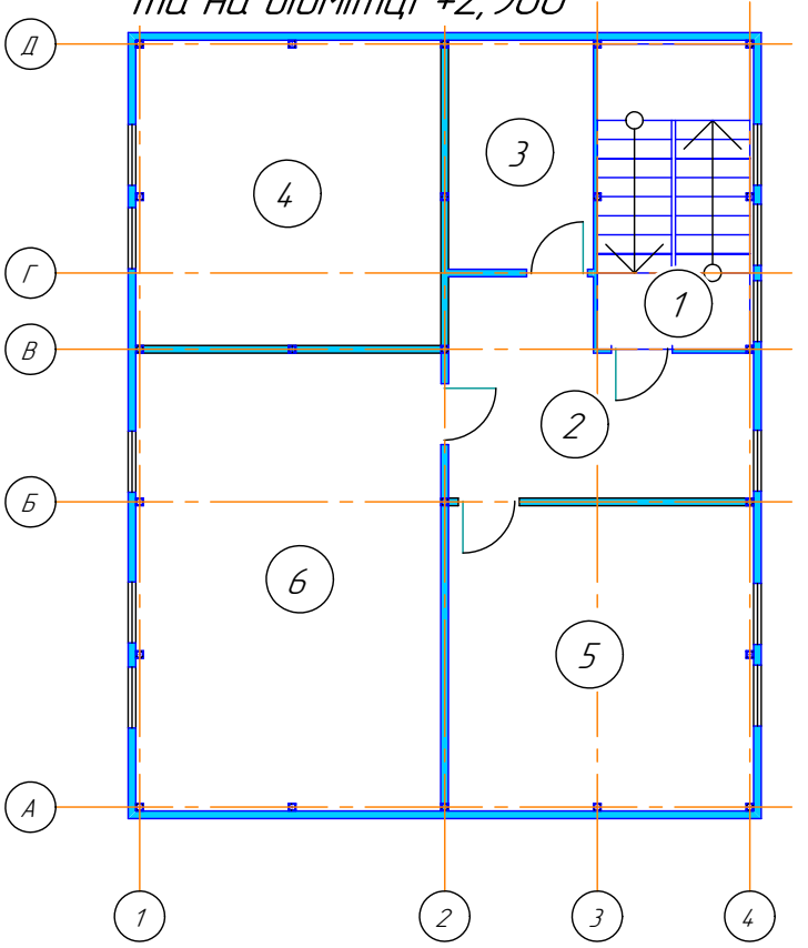
та на відмітці +2,980
