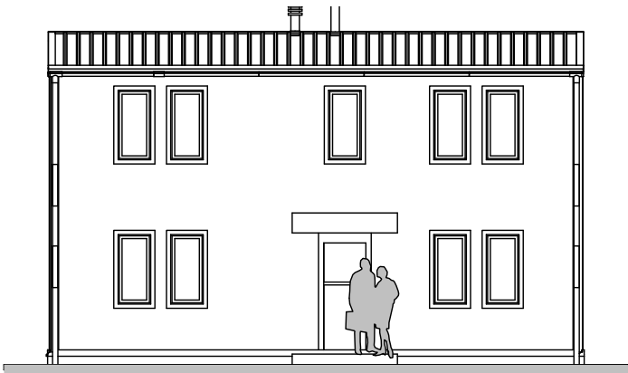
Модель П9 (2-1/8-10/10)
