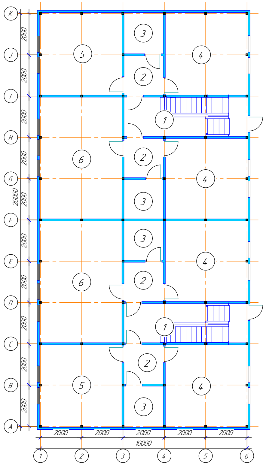
Модель П12 (2-8/2-20/10) План на відмітці 0,000 та на відмітці +2,980
