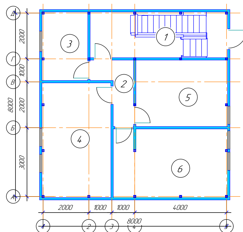
План на відмітці +2,980
