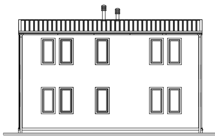
Модель П11 (2-2/4-10/10)
