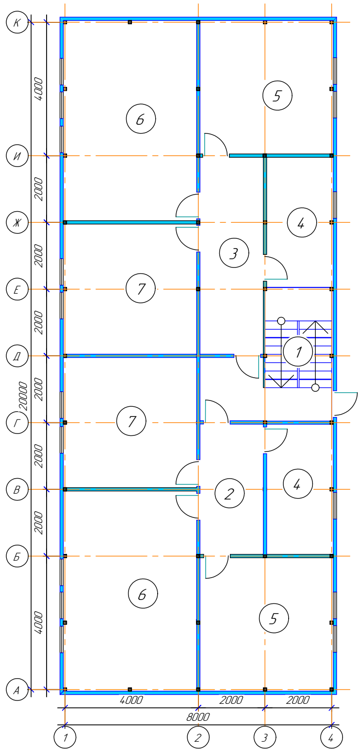
План на відмітці 0,000 та на відмітці +2,980
