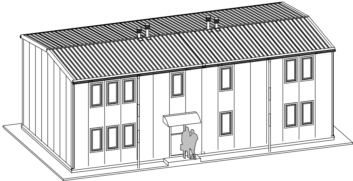
Модель П6 (2-2/2+2/3-16/8)
