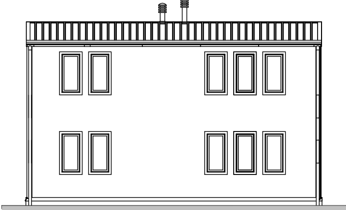
Модель П10 (2-2/3-10/10)
